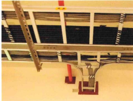
圖 13-明式出線匣及配管
